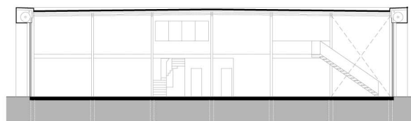
SCHNITT B-B
